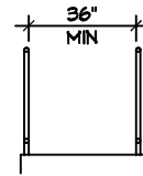
A BARRIER EDGE PROTECTION
