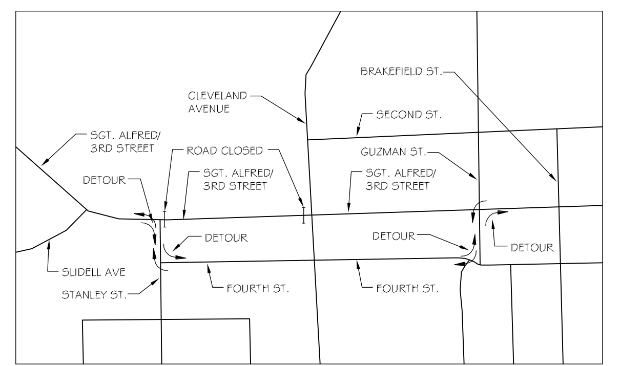
3 DETOUR MAP SCALE: N.T.S.
