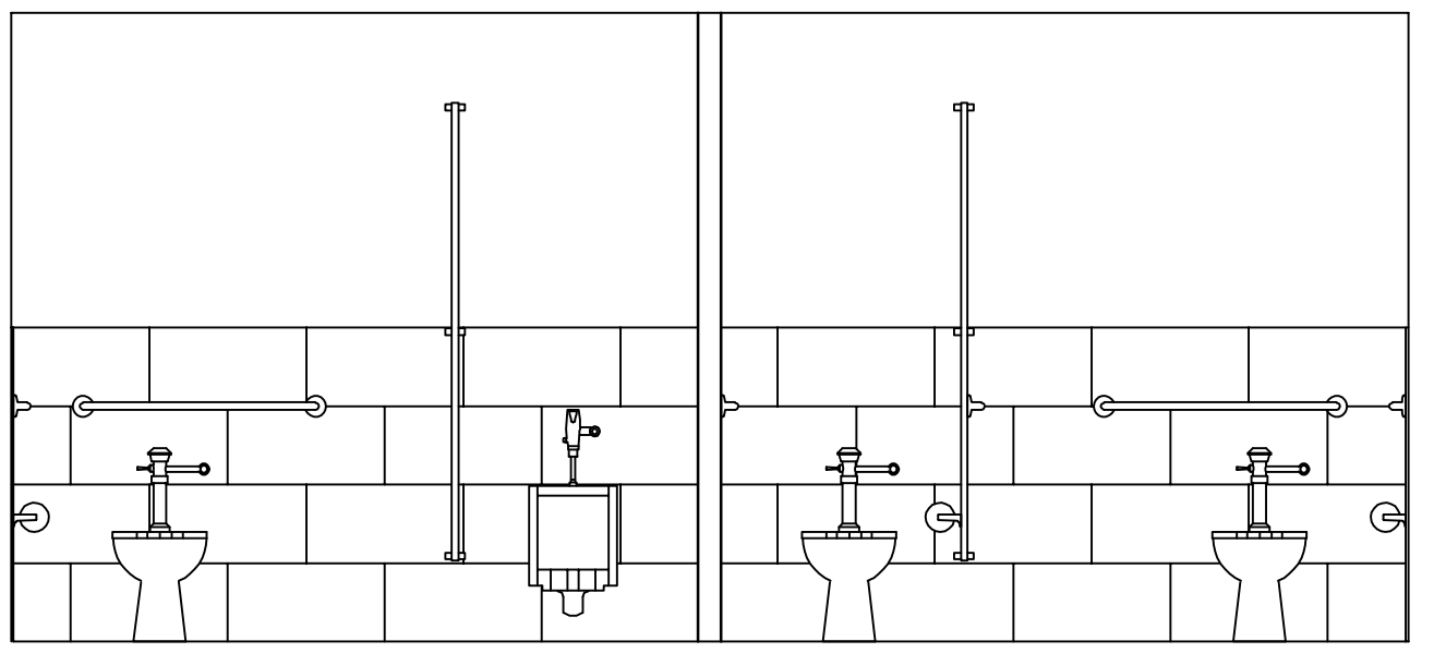
B RESTROOM SCALE: 3/8" = 1'-0"
