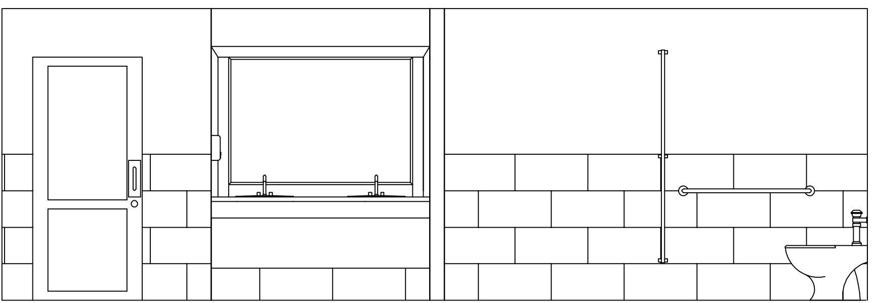
A RESTROOM SCALE: 3/8" = 1'-0"
