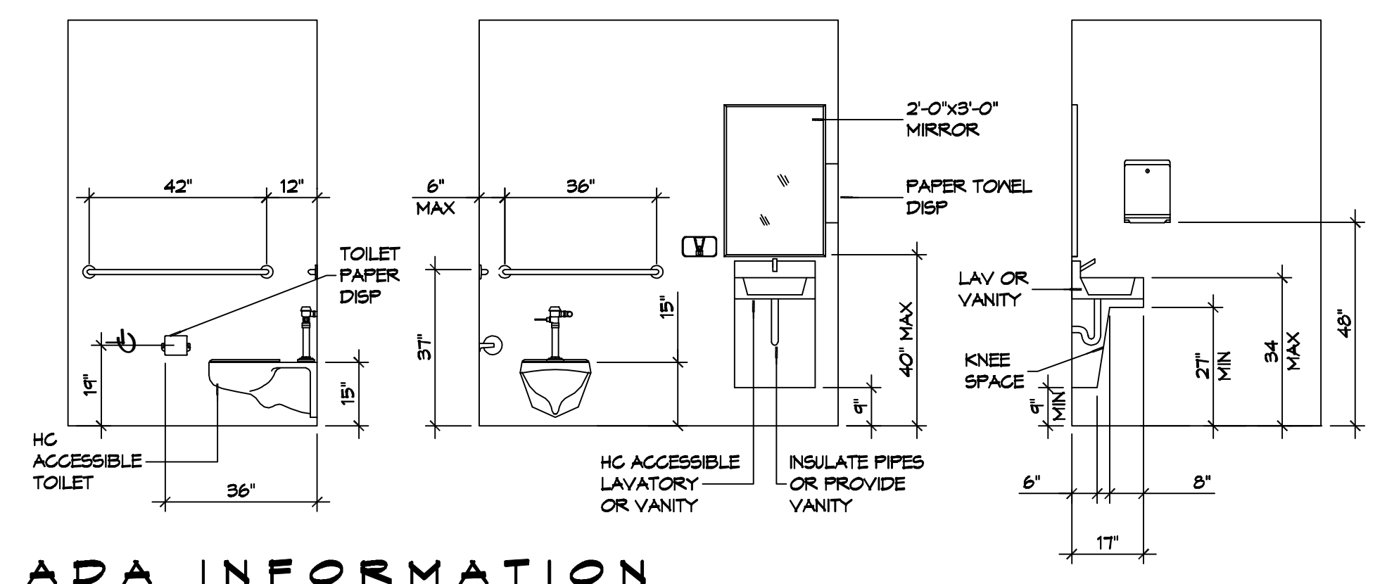
ADA INFORMATION SCALE: 3/8" = 1'-0"
