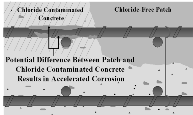
Fig. 1—“Ring-anode” corrosion.
