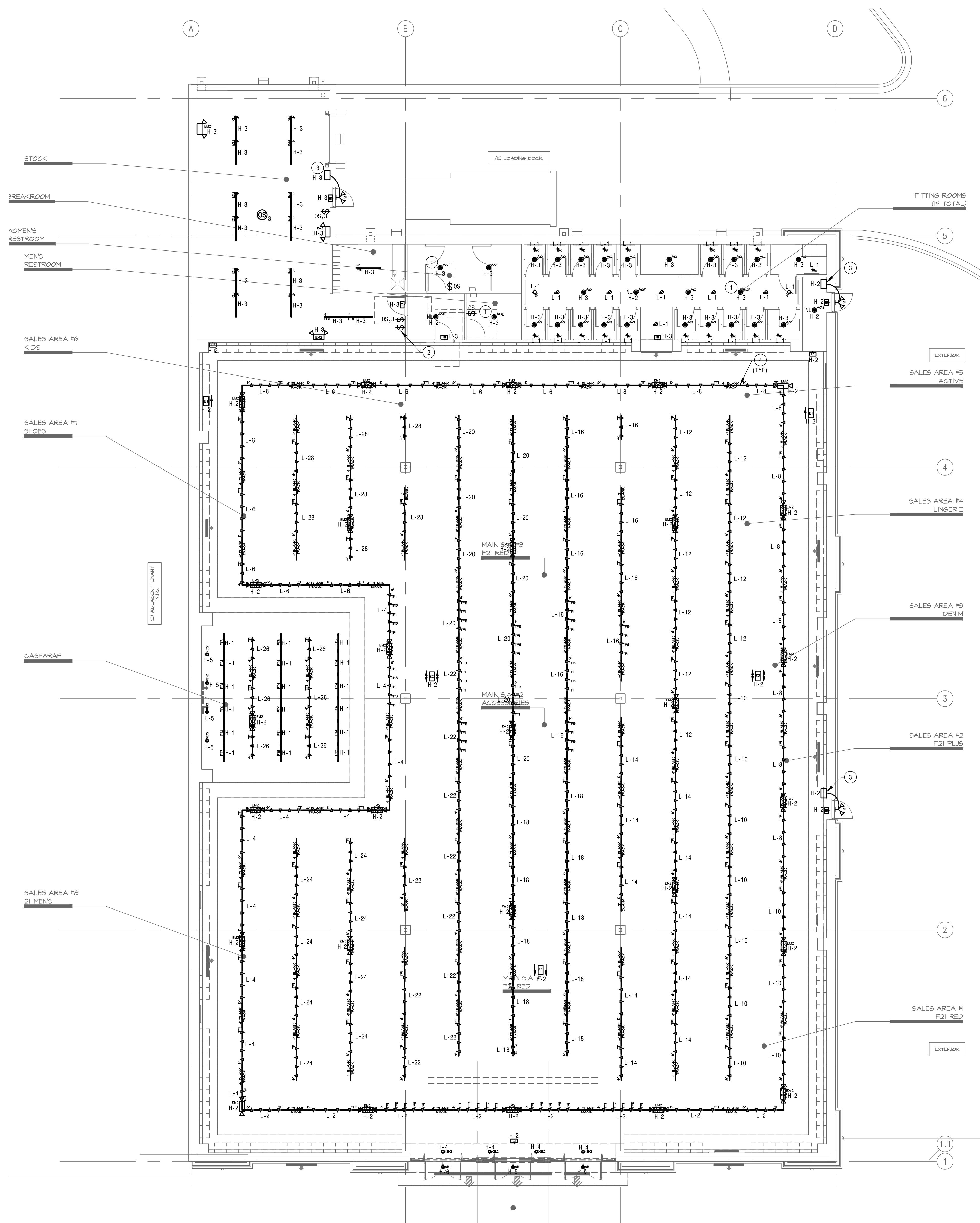
1 LIGHTING PLAN E1.1.0 SCALE: 1/8"=1'-0"
