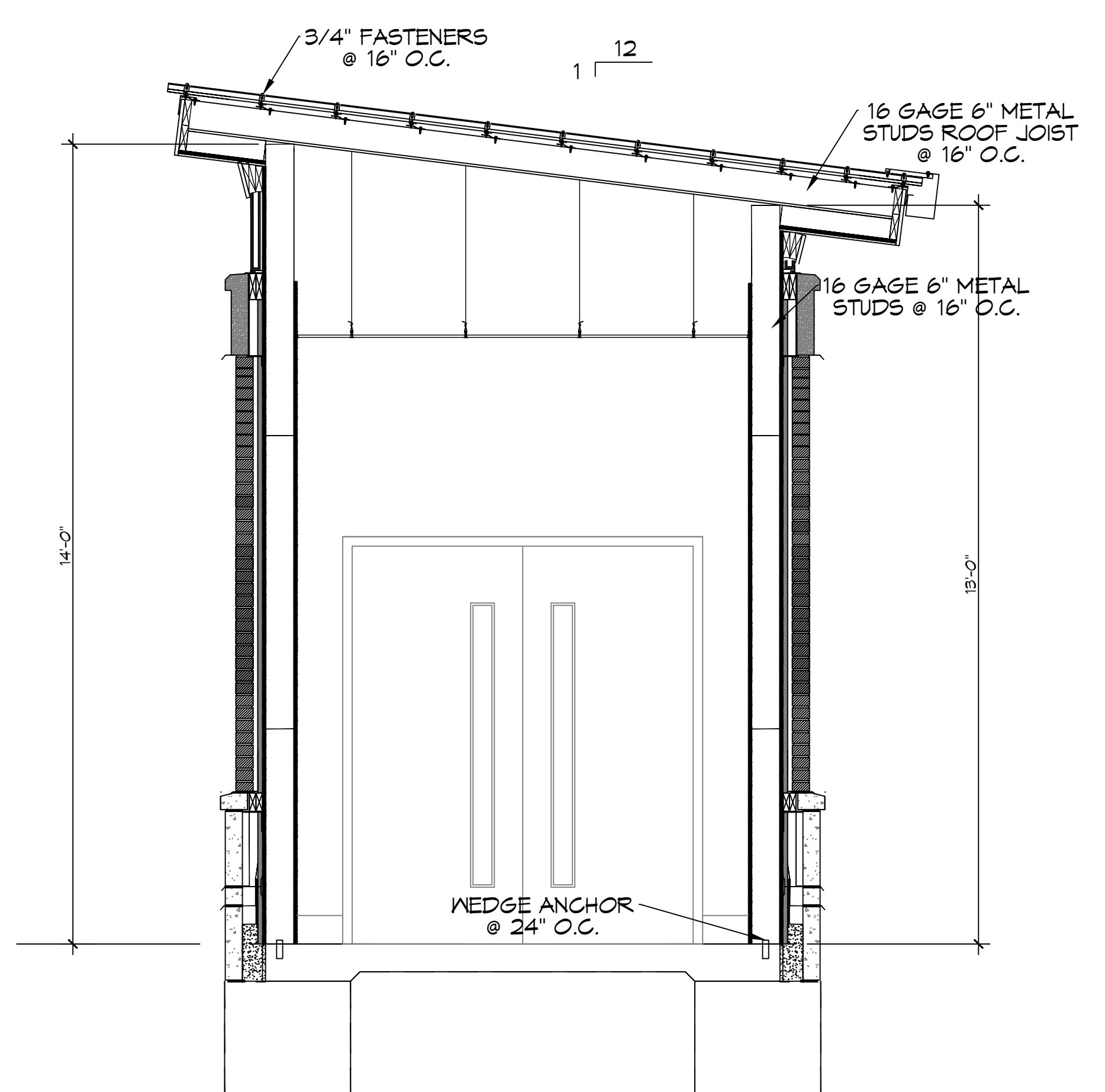
1 SECTION SCALE: 1/2" = 1'-0"
