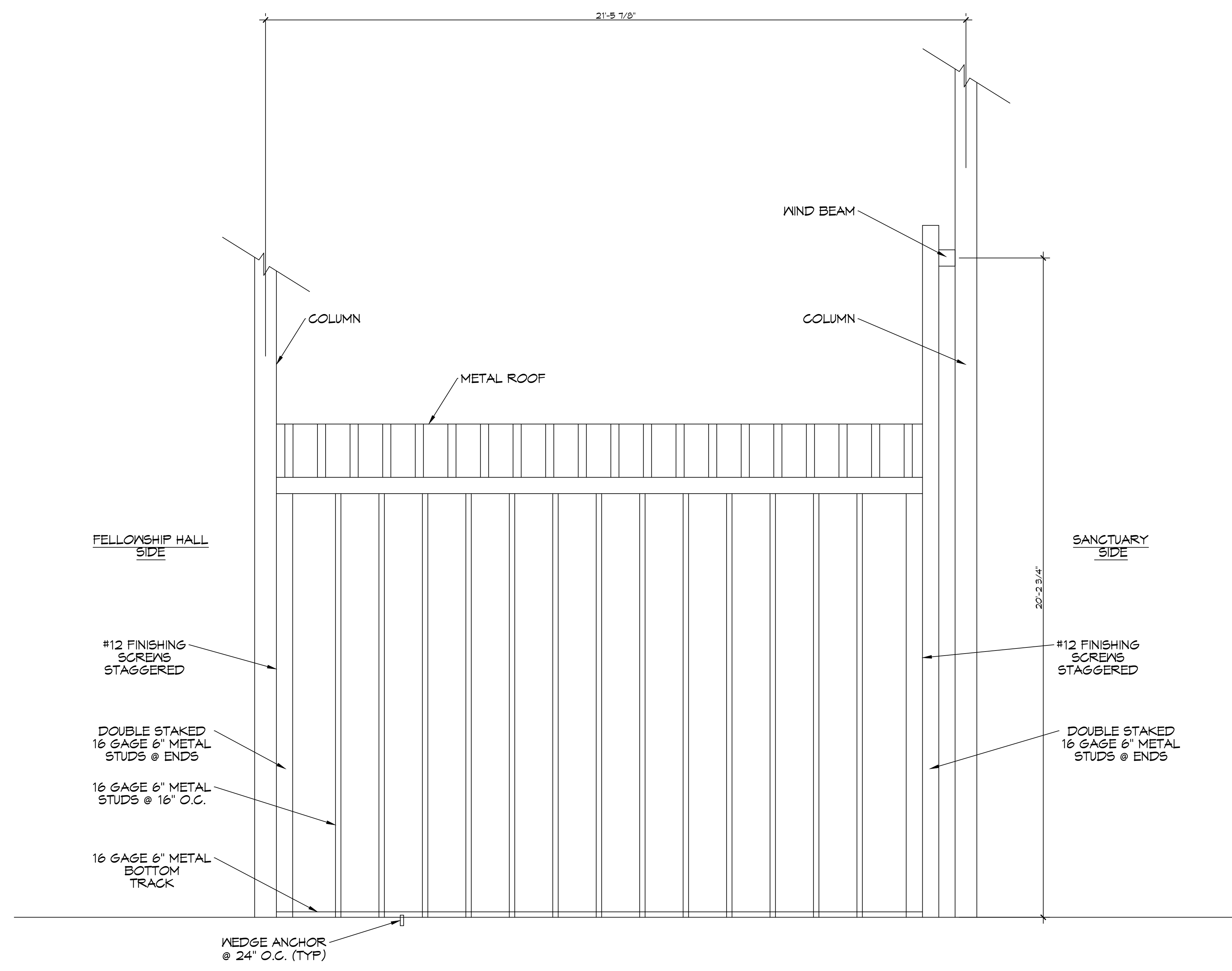
2 SECTION SCALE: 1/2" = 1'-0"
